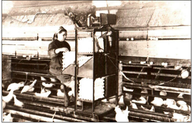
Збір яєць з одночасним сортуванням та частковим пакуванням
