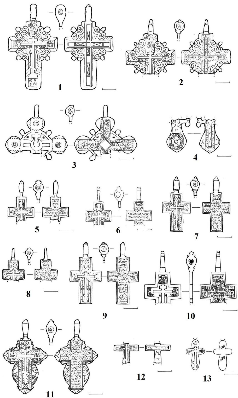
Рисунок 7. Креслення хрестів з території с. Карабінівка (1).
